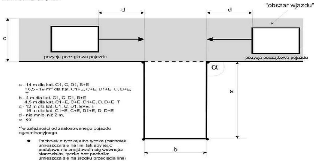
Parkowanie prostopadłe
