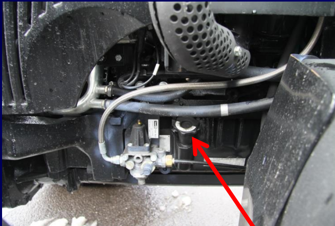
miejsce sprawdzania poziomu oleju
