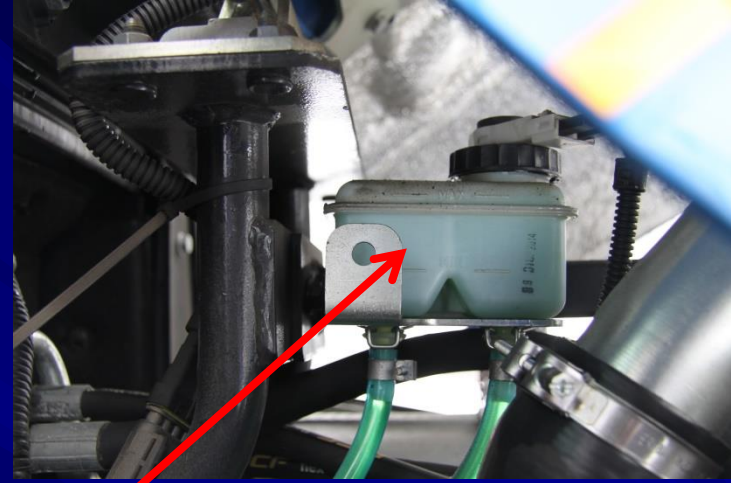
miejsce sprawdzania poziomu płynu hamulcowego
